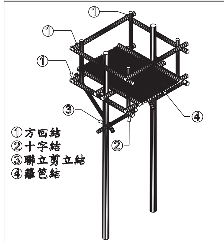
臺北市童軍會高級考驗營工程計畫參考圖說 雙腳瞭望臺
