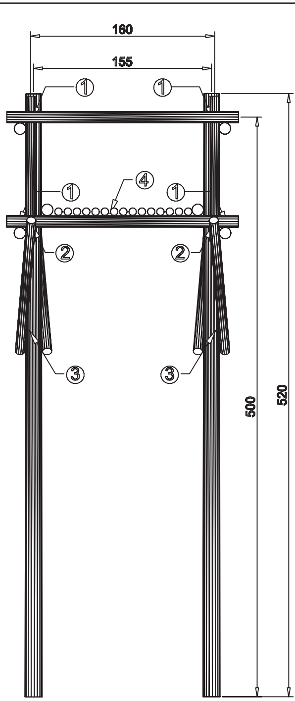
臺北市童軍會高級考驗營工程計畫參考圖說 雙腳瞭望臺
